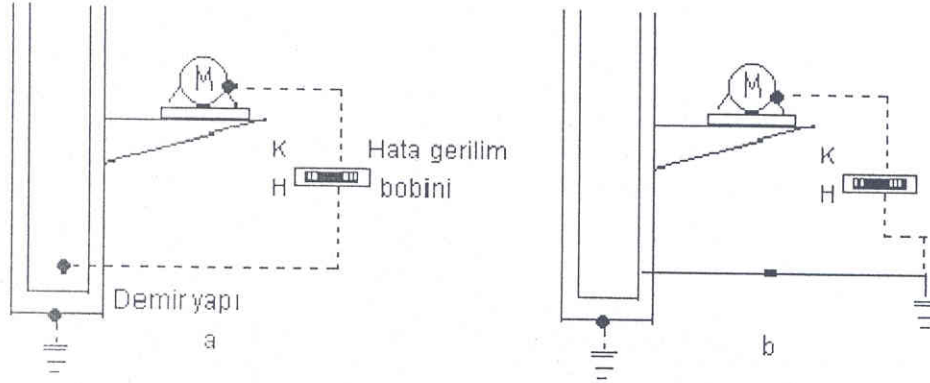
Şekil - 15 Hata gerilimi bobininin bağlanması a İzin verilmeyen bağlanma biçimi b Doğru bağlama biçimi
