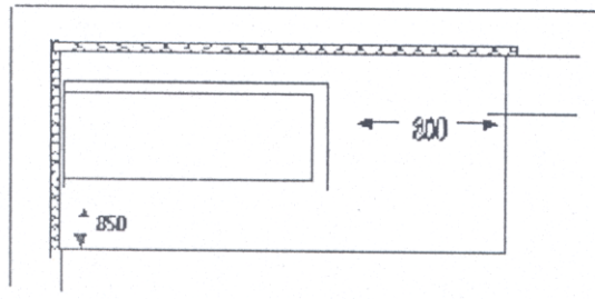
Şekil - 21 Banyoda koruma bölgesi
