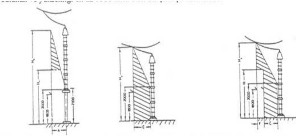
Şekil-5 Dayanak (mesnet) üzerindeki aygıtlarda koruma alanı
